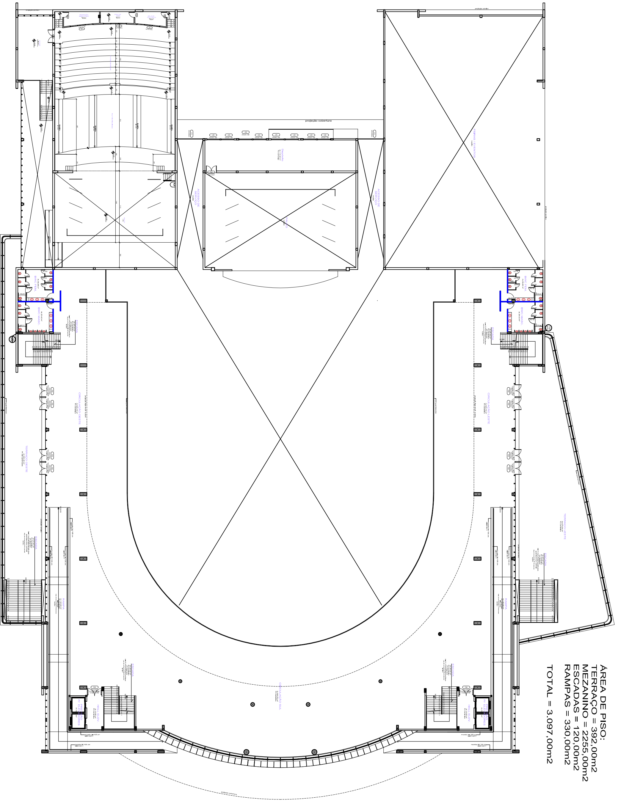
Planta Nivel 4,00 Escala: 1/200
